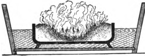
FIG. 131.—Burning Sulphur.
